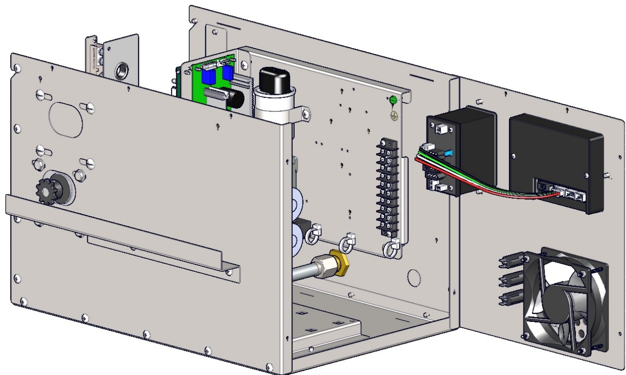
Servisní poloha
